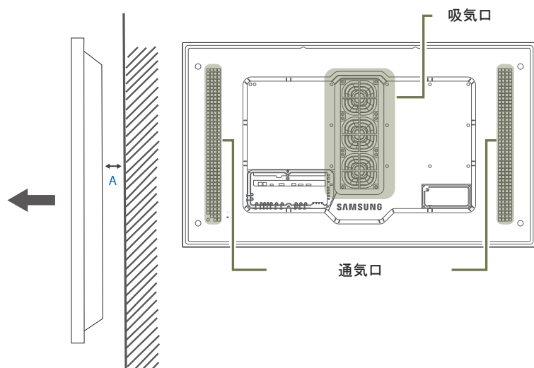
図 1.1 側面図
