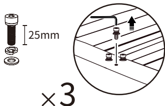
Q M8(25mm) 六角ネジ (座面に付いています)
